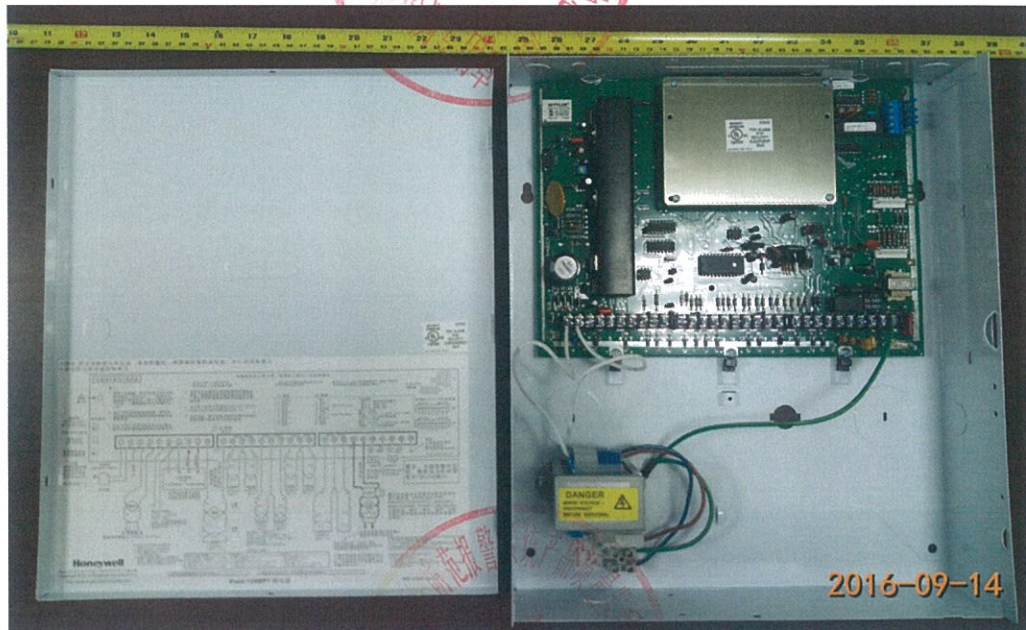
图一、VISTA-128BPT 防盗报警控制主机外部结构
