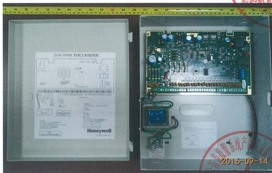
图二、2316 SUPER 防盗报警控制主机内部结构
