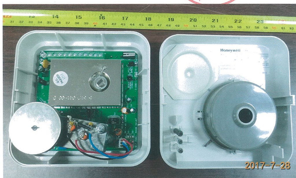
图二、DT-6360STC 微波和被动红外复合报警探测器内部结构
