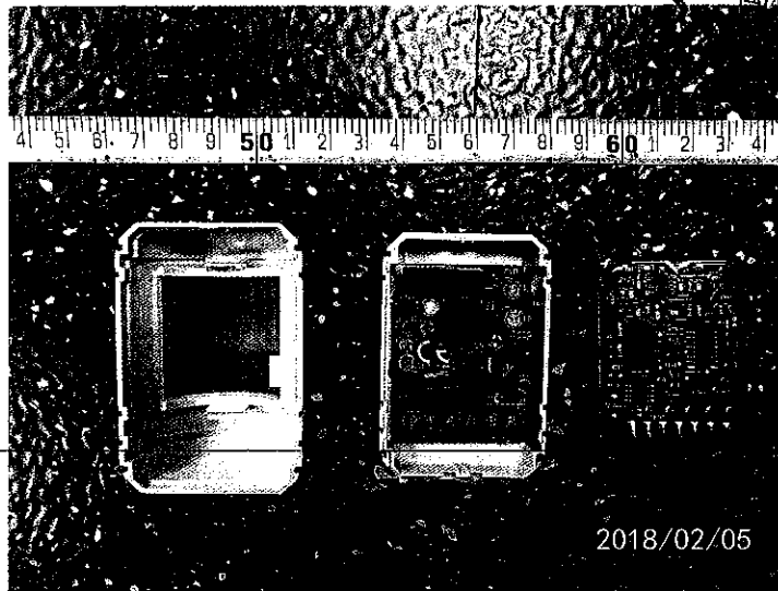
图二、SIR-308P 室内用被动红外探测器内部结构
