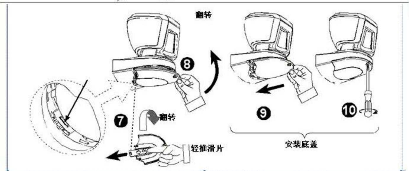
图 4- 距离角度调节及安装底盖
