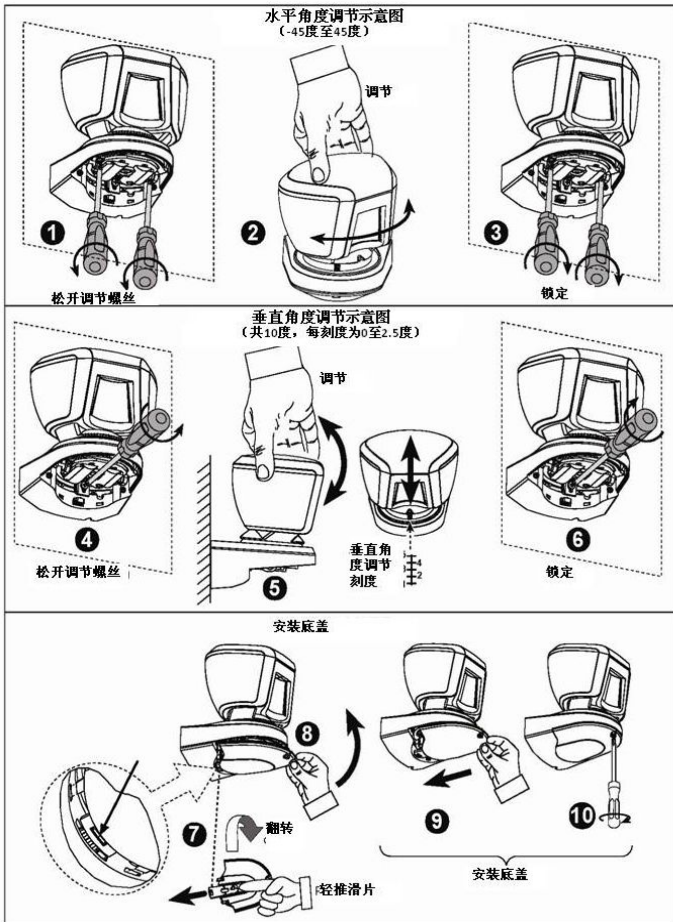
图5 距离调节、安装角度调节
