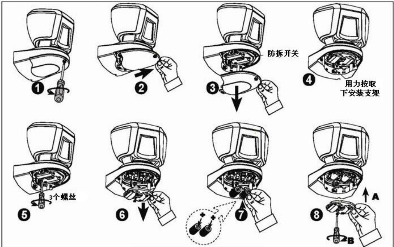
图3 安装电池
