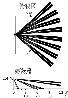
图 2 - 探测区域示意图
