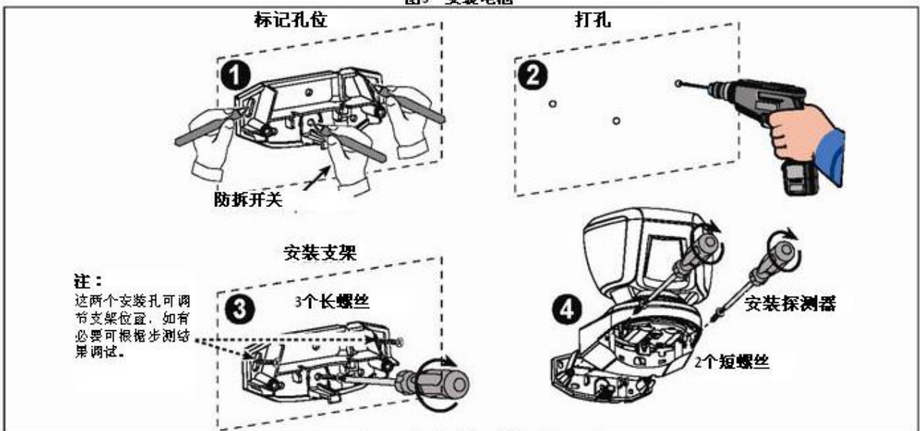
图4 安装支架及探测器
