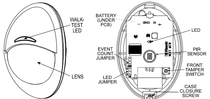
图2. 内部图
