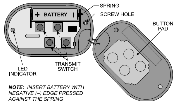
图 2. 取下上盖的内部示意图
