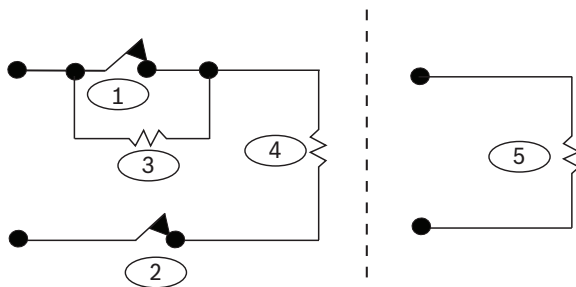
图 12.1: 双 EOL 电阻选件
