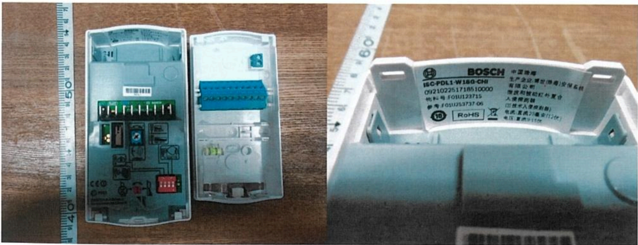
图二: ISC-PDL1-W18G-CHI 型微波和被动红外复合入侵探测器(三技术入侵探测器)内部结构、标识
