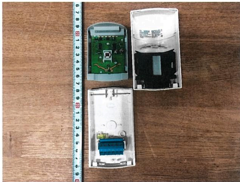
图二: ISC-BDL2-WP6G-CHI 型微波和被动红外复合入侵探测器 (蓝色系列 G2 三技术防宠物入侵探测器) 内部结构
