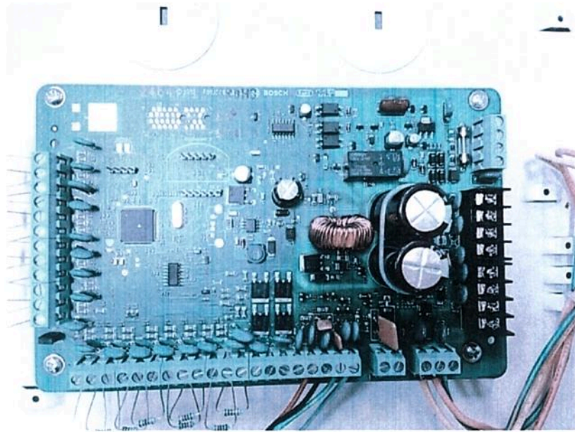
图三: ICP-CMS40-CHI 防盗报警控制器(CMS 系列)主板结构
