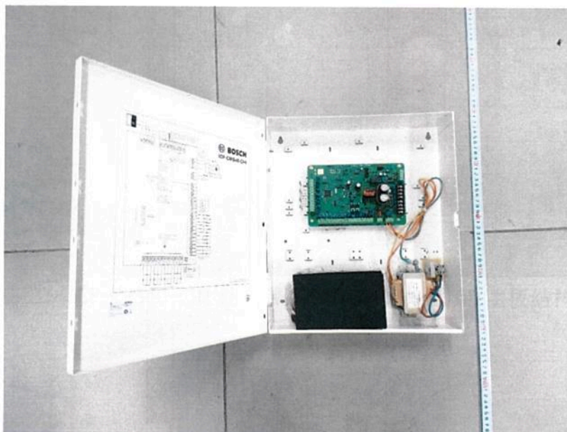
图二： ICP-CMS40-CHI 防盗报警控制器 (CMS 系列) 主机内部结构
