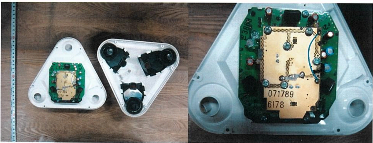
图二: DS9370-CHI 型吸顶式三技术入侵探测器 (微波与被动红外复合入侵探测器) 内部结构
