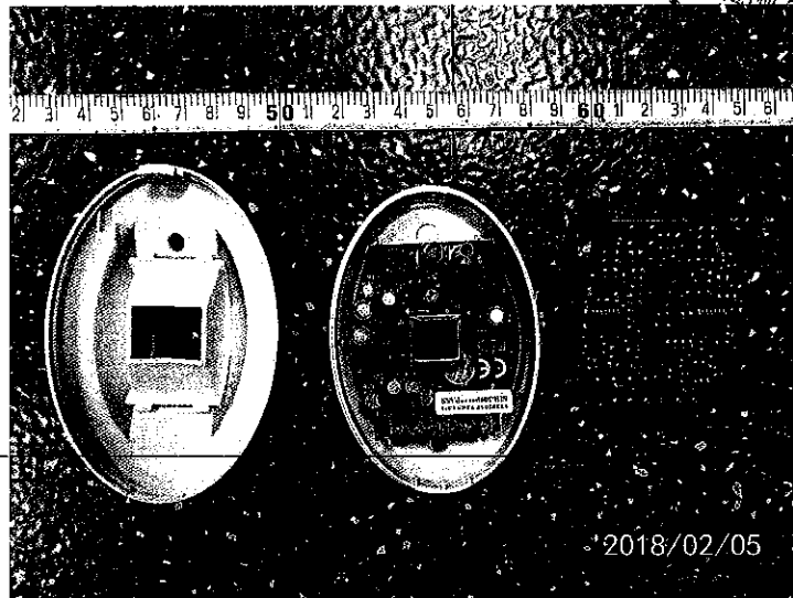
图二、SIR-309P 室内用被动红外入侵探测器内部结构
