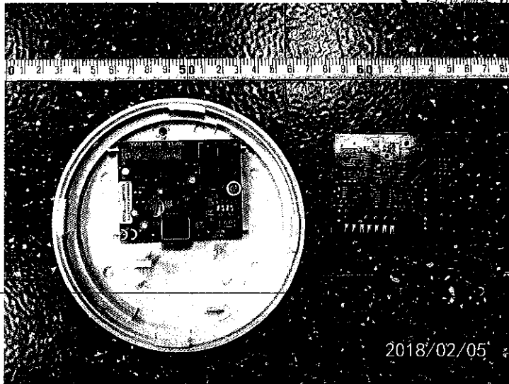
图二、SIR-306P 室内用被动红外入侵探测器内部结构
