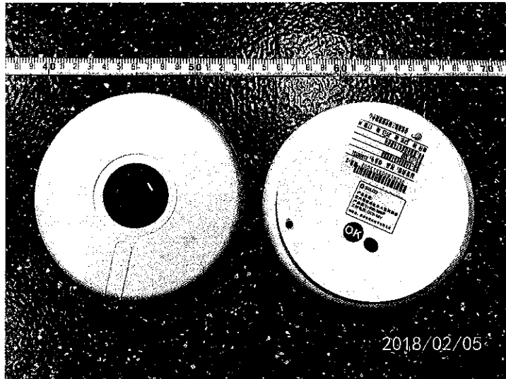
图一、SIR-306P 室内用被动红外入侵探测器外部结构
