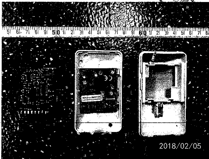
图二、RK210PR 室内用被动红外探测器内部结构
