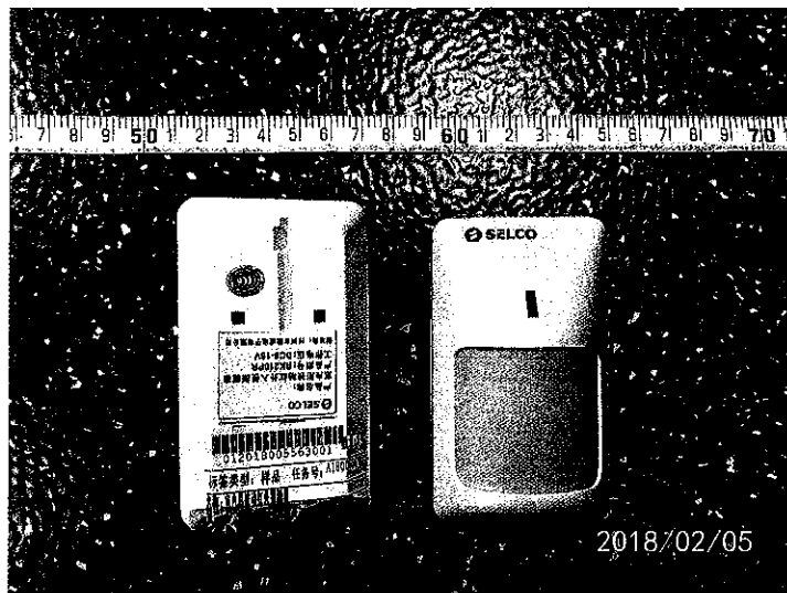
图一、RK210PR 室内用被动红外探测器外部结构
