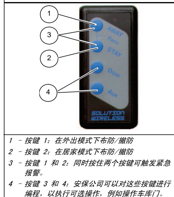
图 4: RE013/E: 4 通道无线密钥发射器
