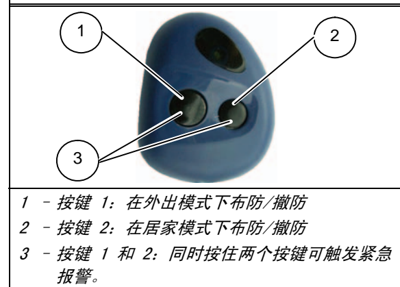
图 3: RE012/E: 双通道无线密钥发射器
